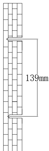
Fig. 4-B: Instalación invertida
