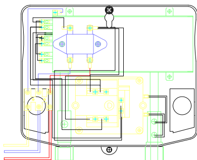
Fig. 5-A: Instalación vertical común
